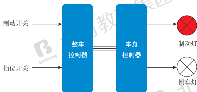
图 1 制动灯和倒车灯控制逻辑图
