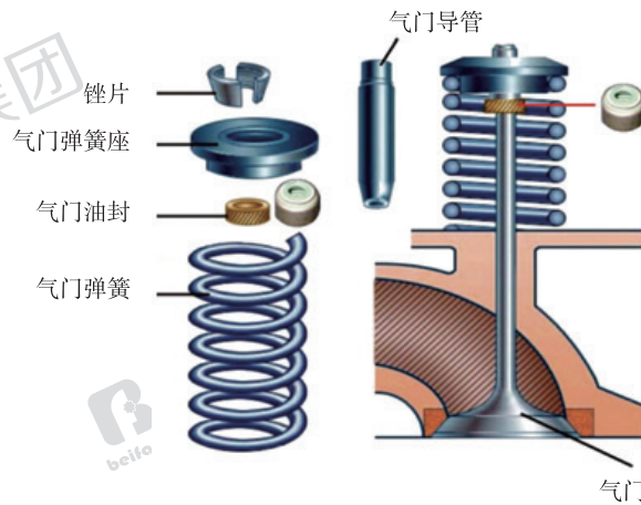
图 1 气门组
