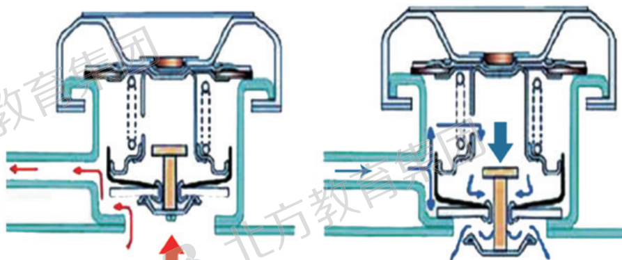
图 1 水箱盖
