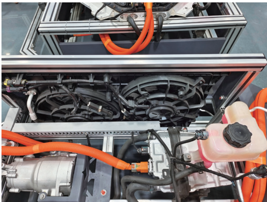
图 2-1-13 散热风扇与冷凝器
