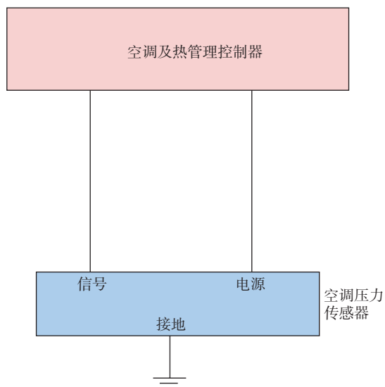
图 5-1-12 空调压力传感器
