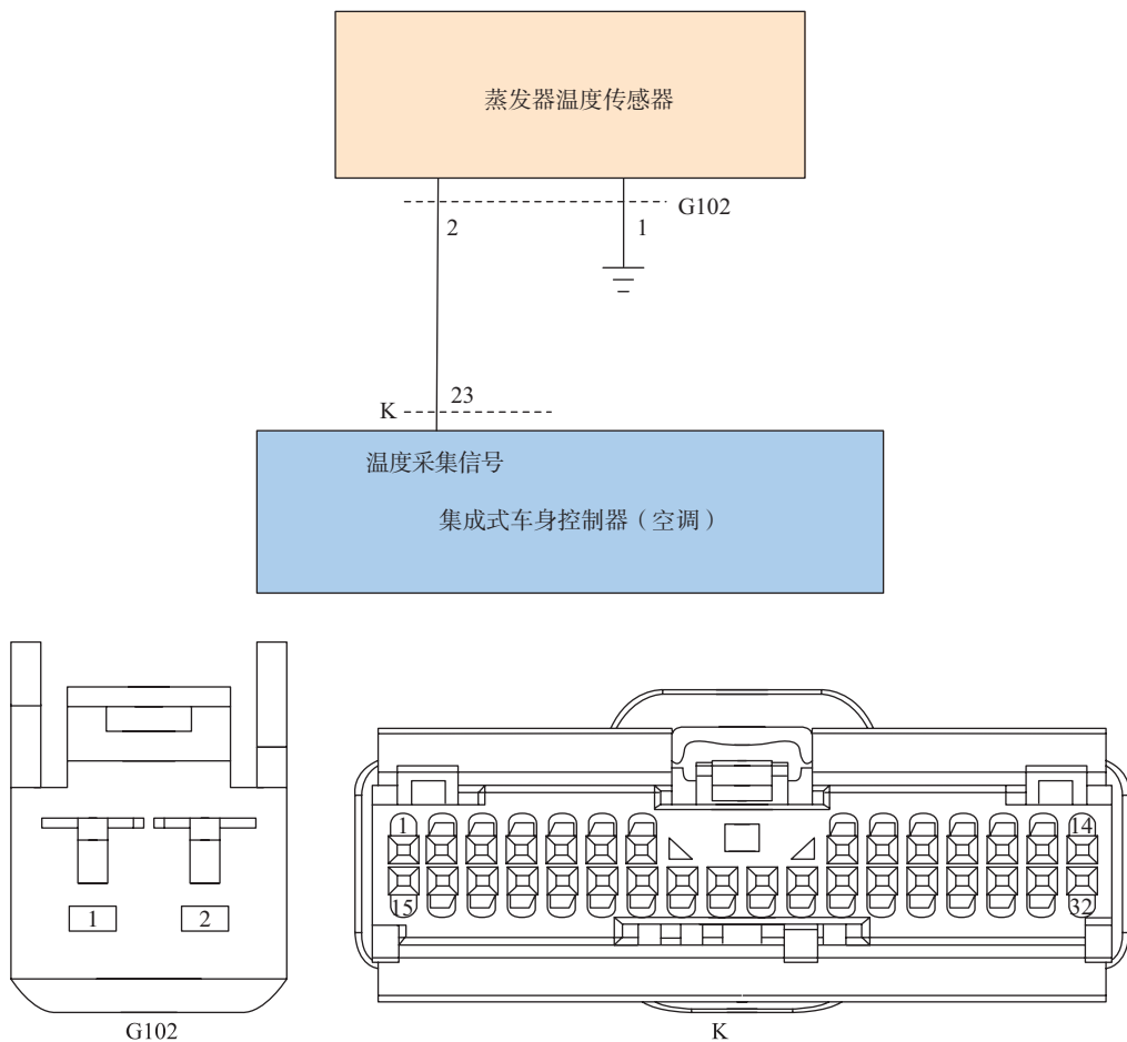
图 5-1-8 秦 PLUS EV 蒸发箱温度传感器电路及相关端子
