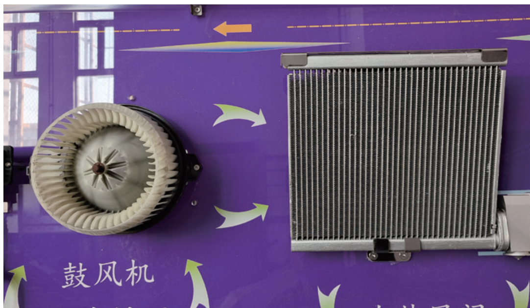
图 2-3-12 鼓风机与蒸发箱
