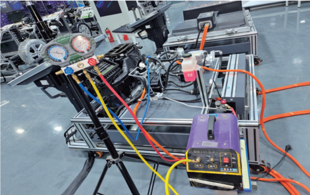
图 2-6-8 连接真空泵
