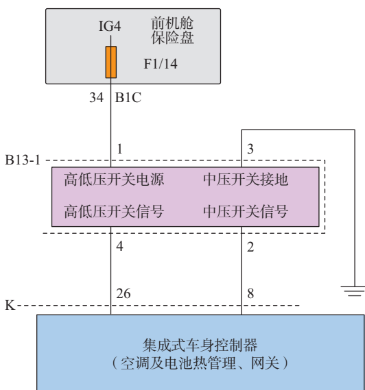
图 2-3-5 秦 PLUS EV 空调压力开关电路
