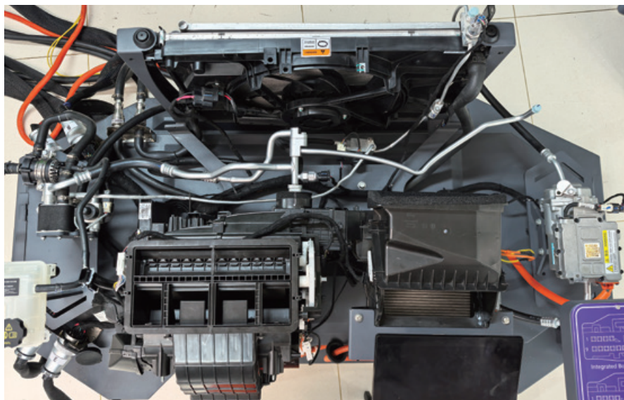
图 2-5-5 秦 PLUS EV 空调制冷系统组成
