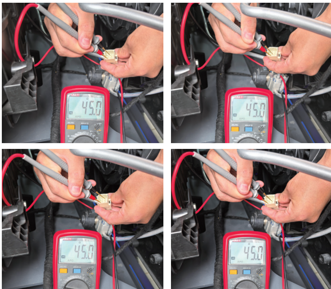
图 2-4-16 电子膨胀阀阻值测量
