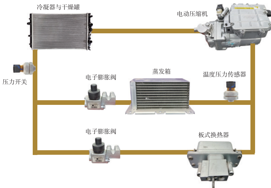
图 2-5-3 秦 PLUS EV 空调制冷系统图
