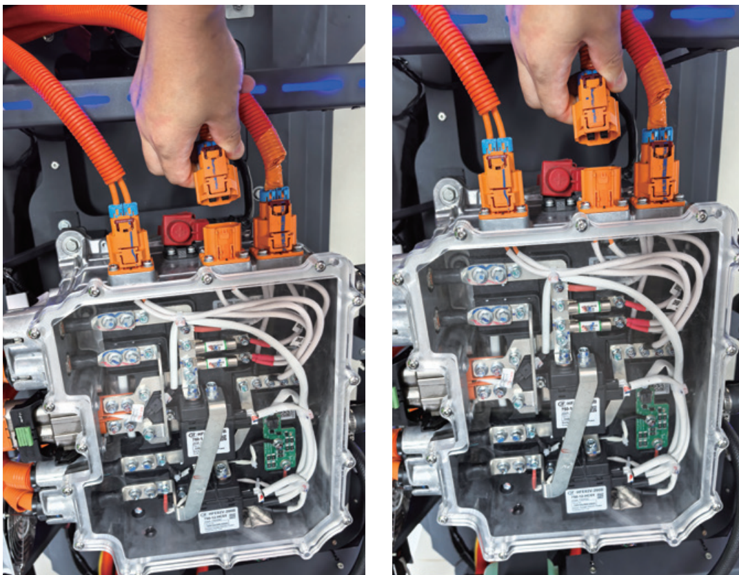
图 2-2-8 拔下电动压缩机的高压插头
