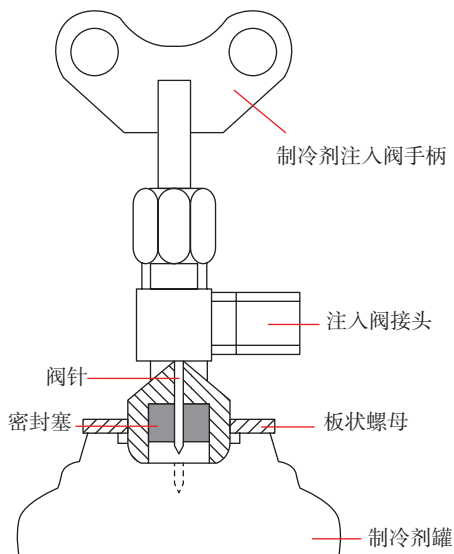
图 2-6-3 制冷剂充注阀
