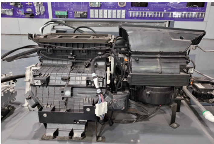
图 4-2-1 空调配气系统
