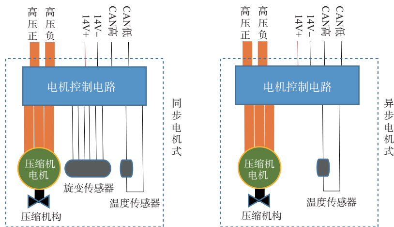
图 2-2-3 电动压缩机电路
