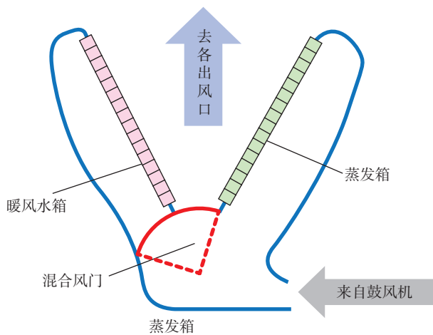
图 5-2-6 温度调节旋钮冷端时冷暖空气混合风门位置
