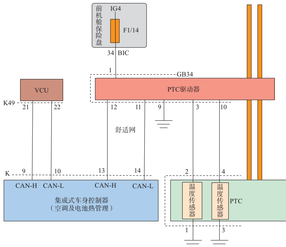
图 3-1-9 秦 PLUS EV PTC (空调) 控制电路
