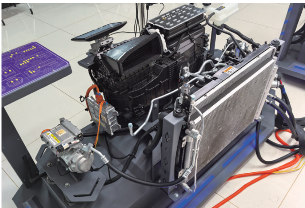
图 2-3-2 冷凝器的位置
