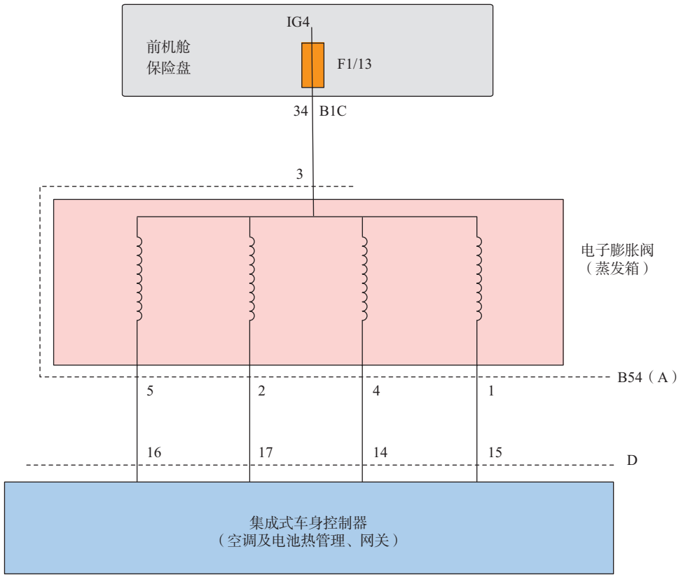
图 2-4-11 秦 PLUS EV 电子膨胀阀控制电路
