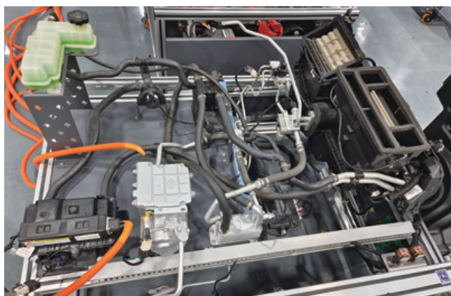
图 1-21 电动压缩机与 PTC
