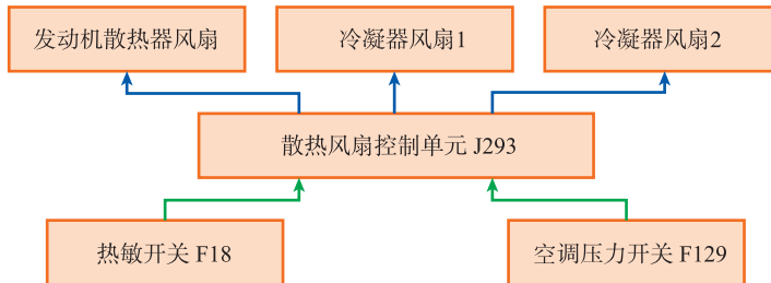
图 2-3-10 双电机串并联式散热风扇控制电路
