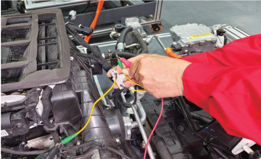
图 4-2-21 出风模式风门伺服电机通电实验（转向吹面端）
