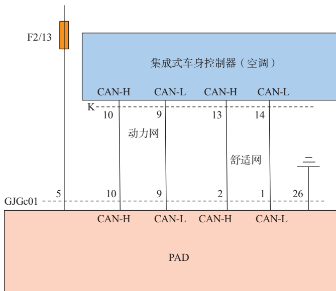
图 5-2-16 秦 PLUS EV 液晶控制屏电路
