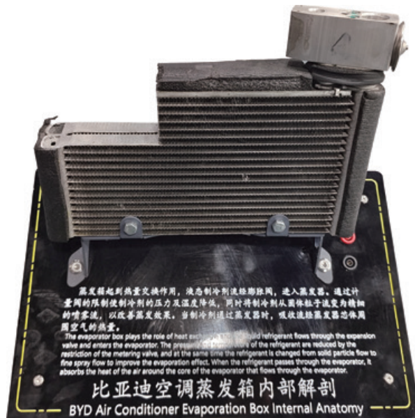
图 2-1-10 蒸发箱
