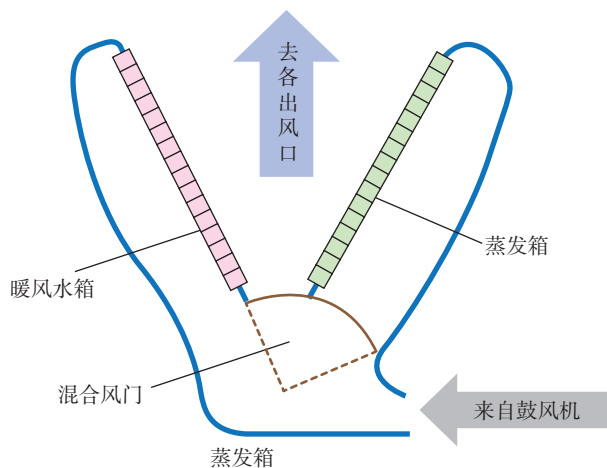
图 4-2-8 秦 PLUS EV 冷暖控制混合段结构示意图
