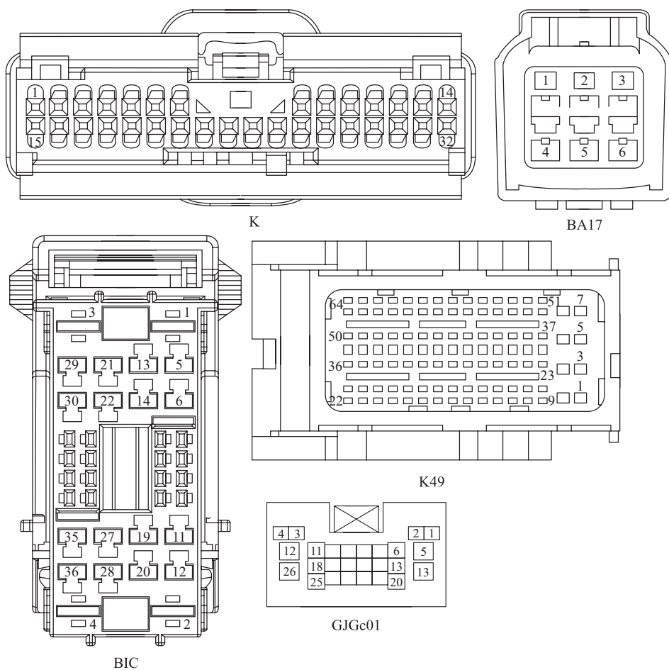
图 2-2-5 电动压缩机相关插头
