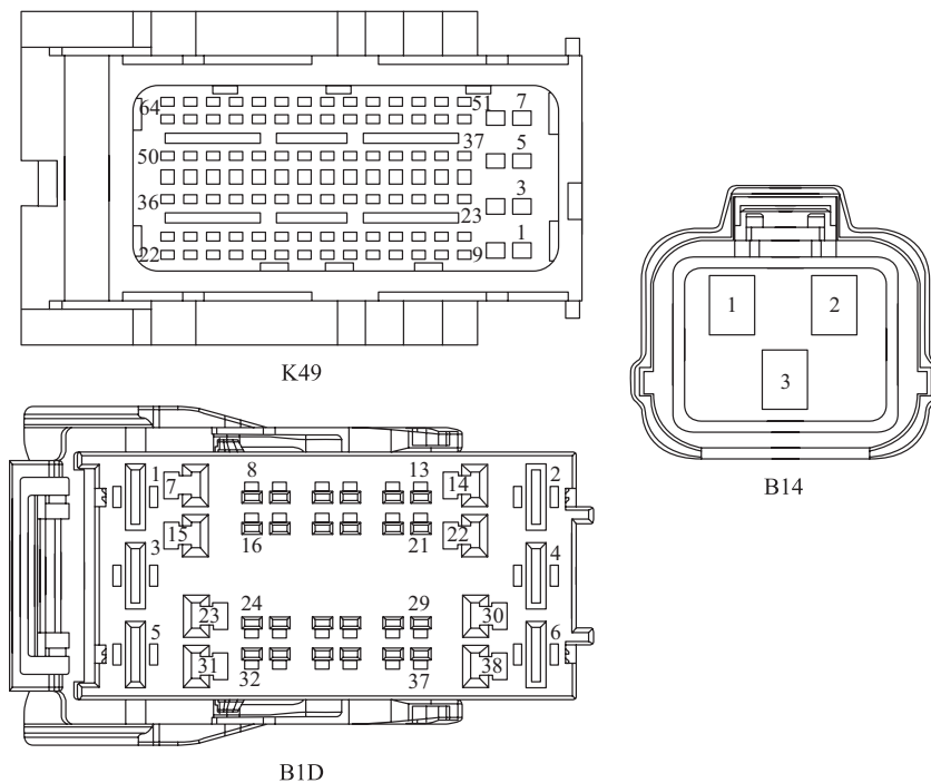
图 2-3-8 前舱保险盒插头
