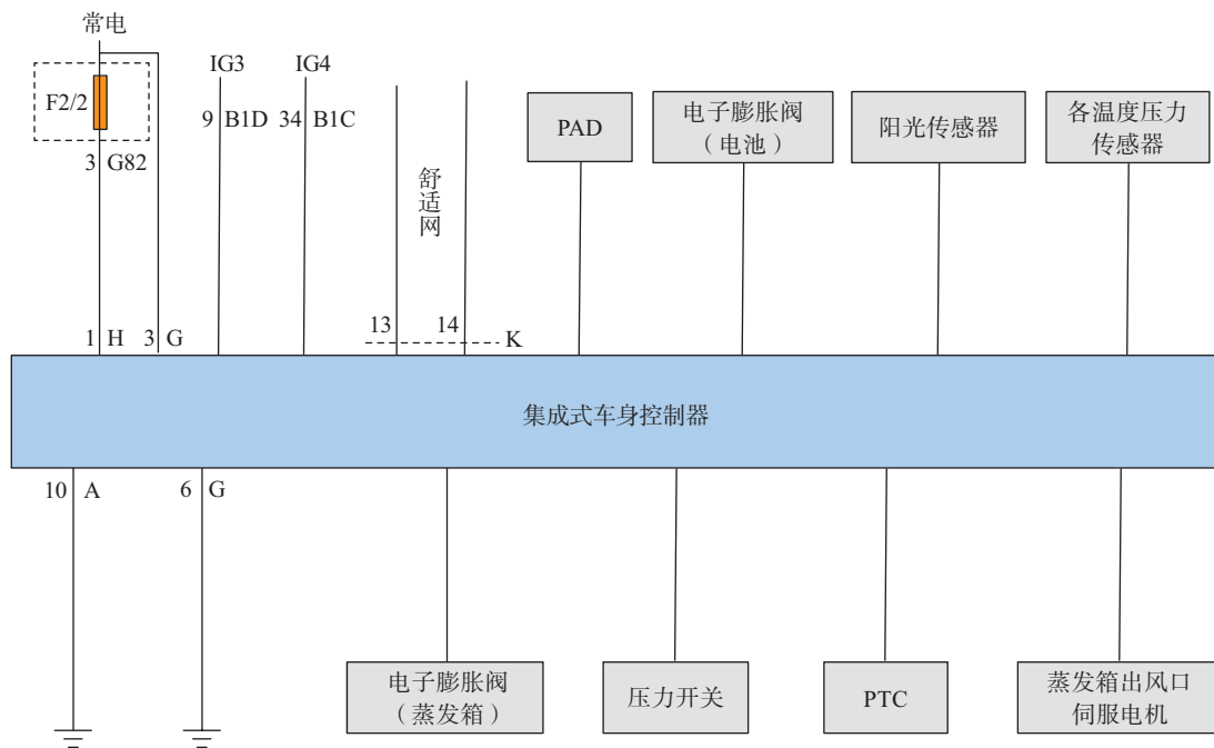
图 5-3-9 秦 PLUS EV 空调控制电路
