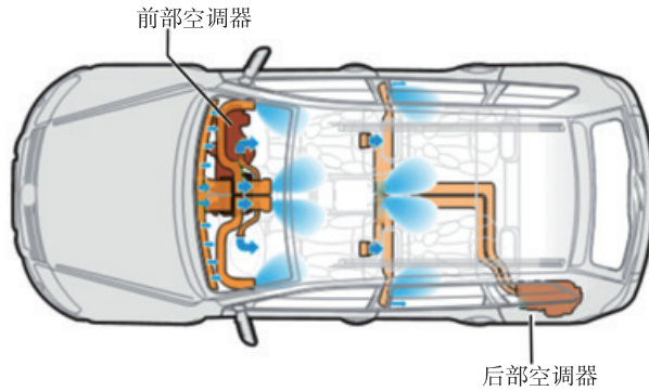
图 5-3-6 前后空调器
