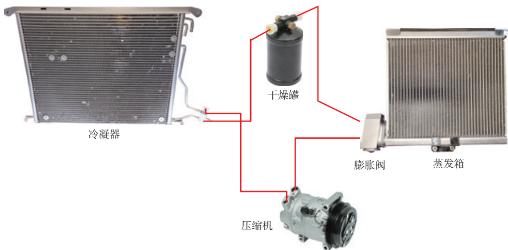
图 2-1-8 汽车制冷系统的组成
