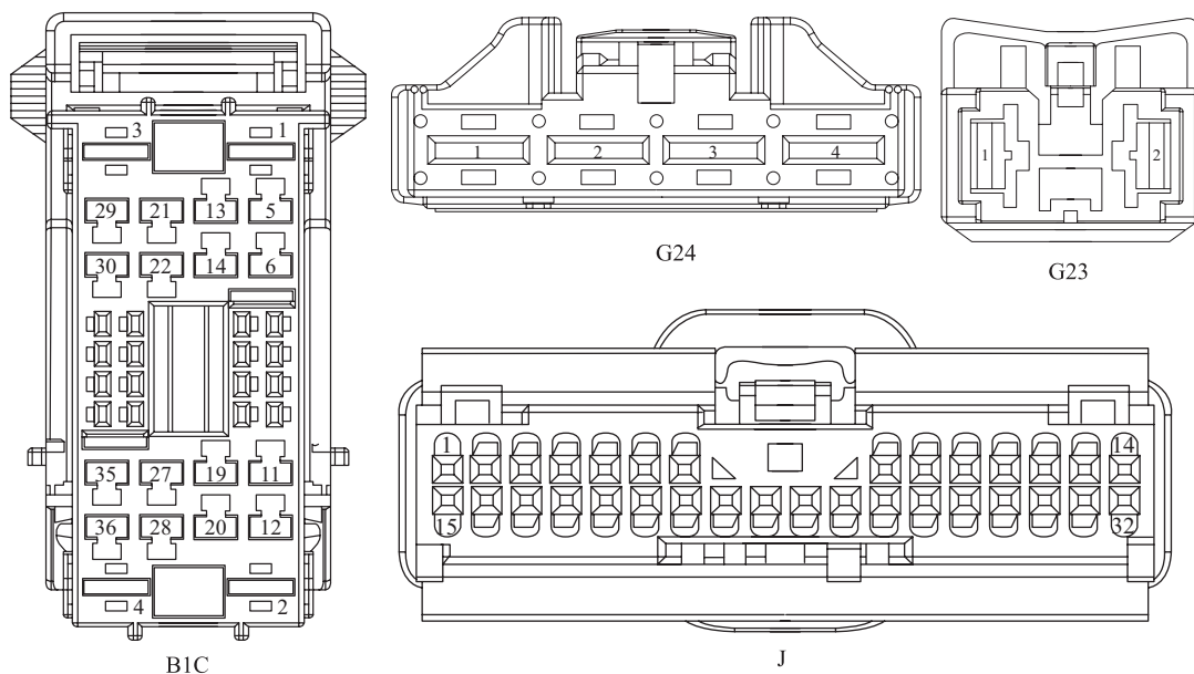
图 2-3-19 鼓风机相关插头
