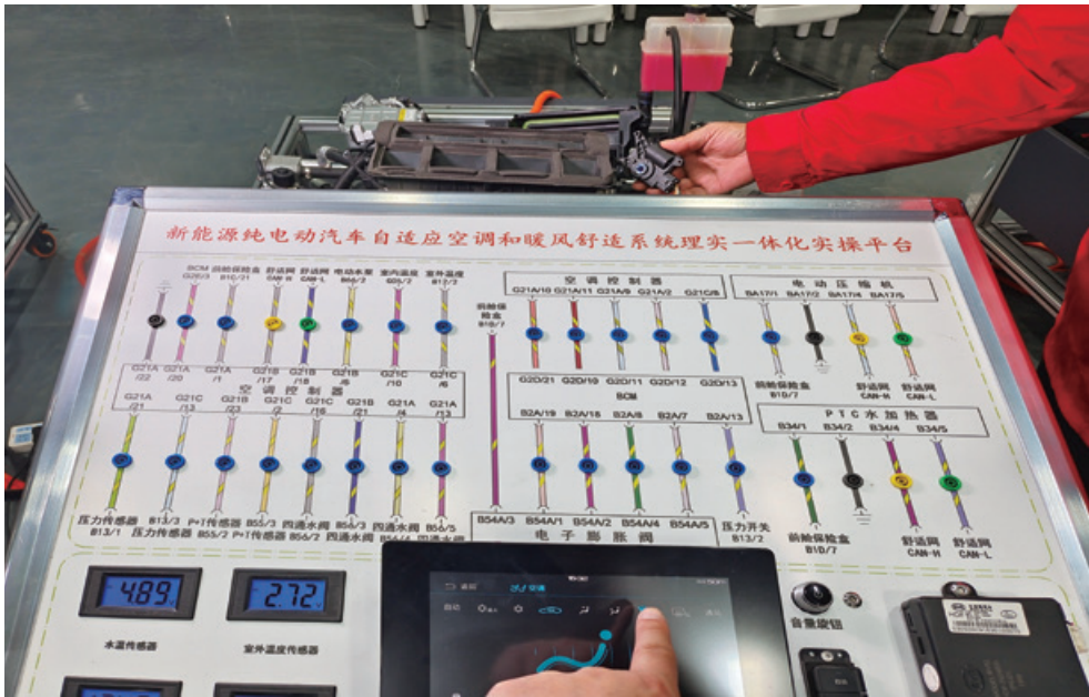
图 4-2-19 调整伺服电机
