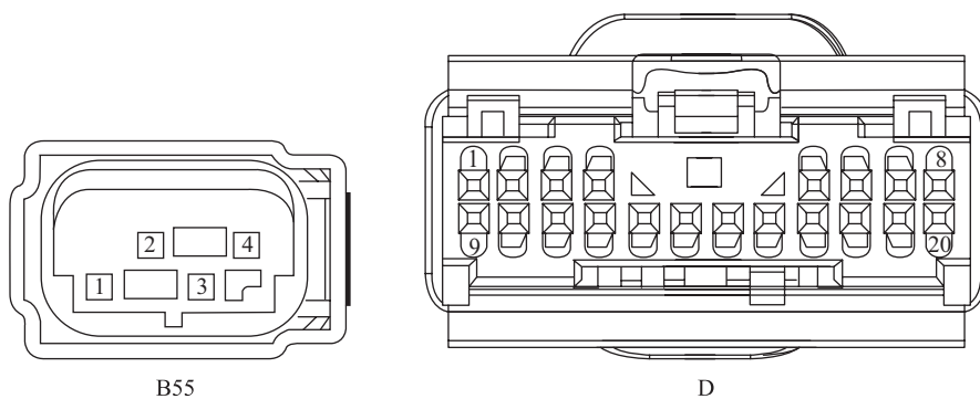
图 2-4-15 秦 PLUS EV 温度压力传感器相关插头
