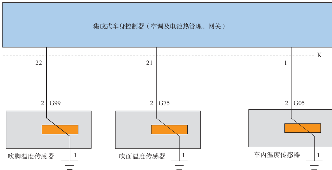
图 5-1-4 秦 PLUS EV 各车内温度传感器电路
