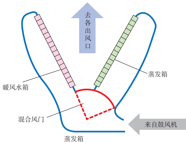
图 5-2-7 温度调节旋钮热端时冷暖空气混合风门位置
