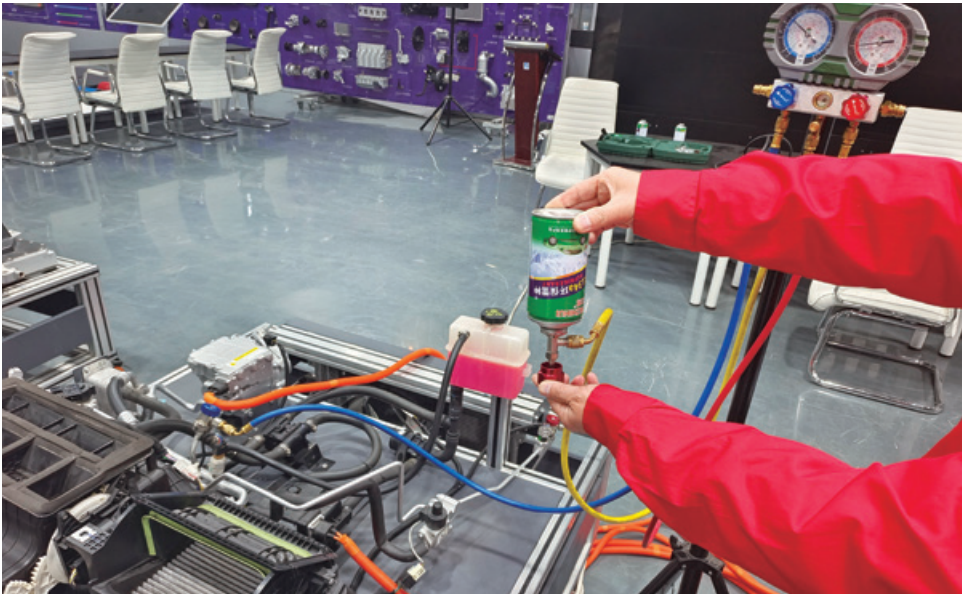
图 2-6-12 高压侧充入液态制冷剂（制冷剂罐倒立）
