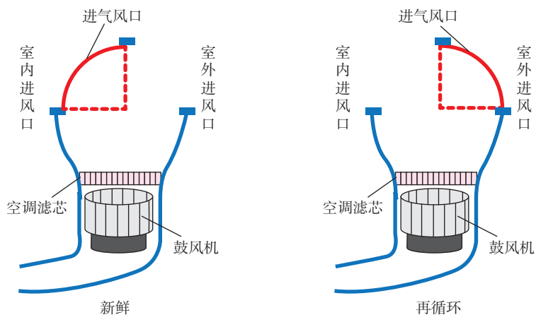
图 4-2-5 进气风门的位置
