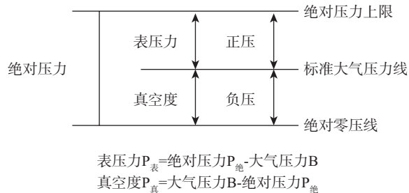
图 2-6-4 绝对压力和表压力与真空度的关系
