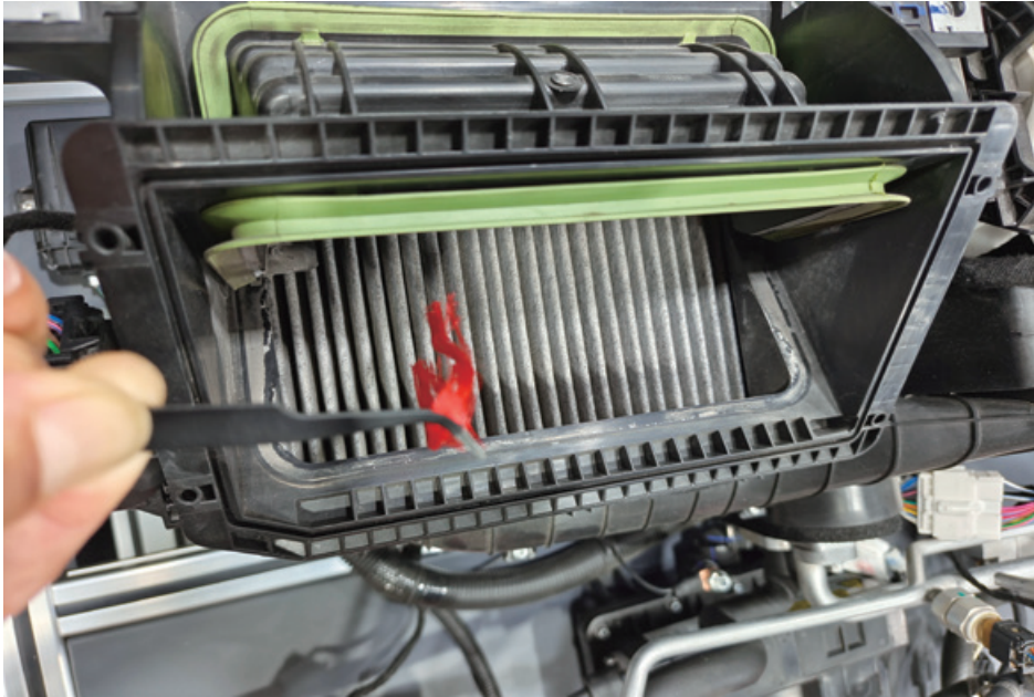
图 4-1-10 进风口的空气流动
