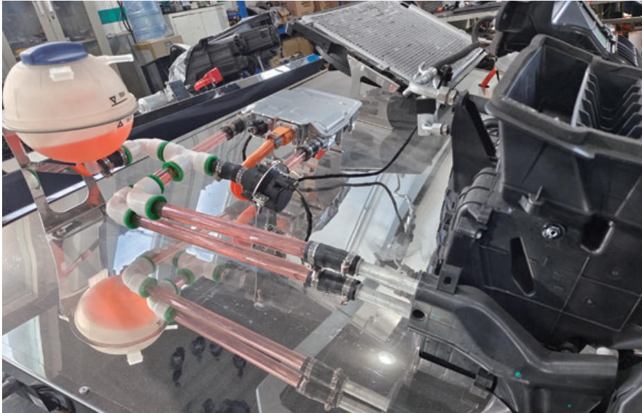
图 3-1-5 电动汽车暖风系统
