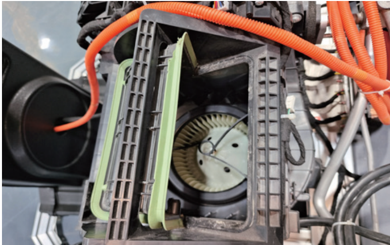
图 4-2-7 秦 PLUS EV 鼓风机
