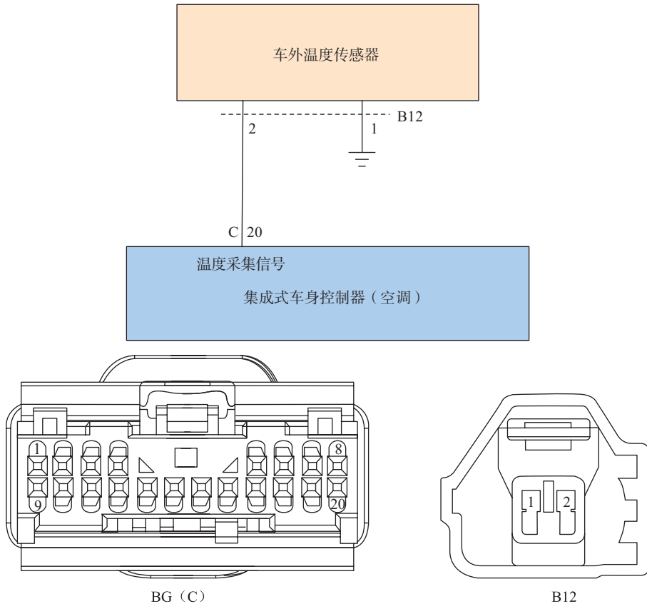
图 5-1-7 秦 PLUS EV 车外温度传感器电路及相关端子
