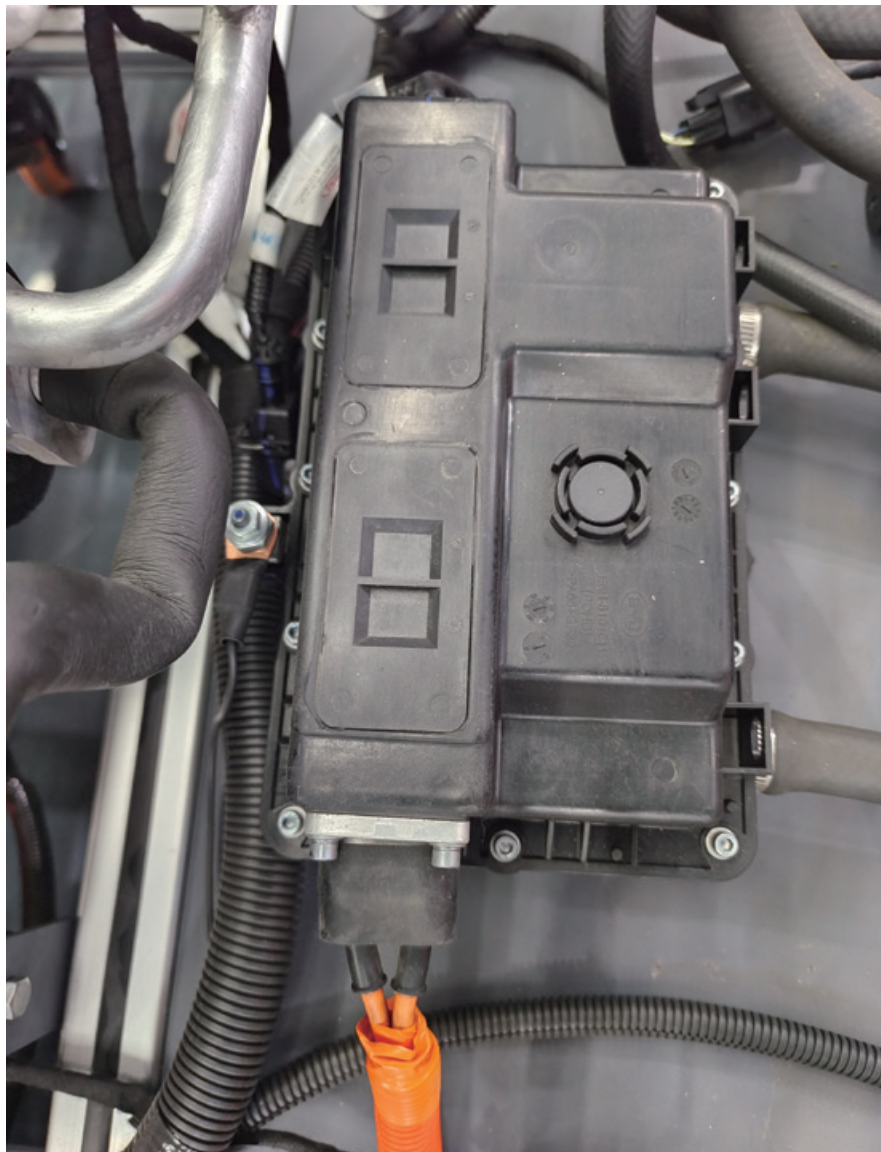
图 3-1-4 秦 EV PTC
