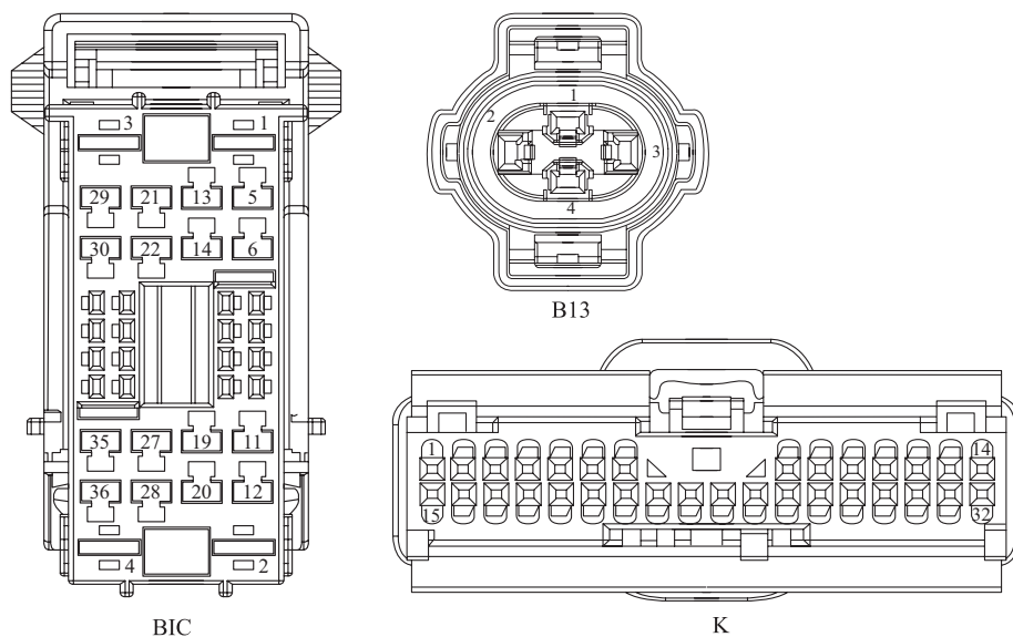
图 2-3-6 秦 PLUS EV 空调压力开关插头
