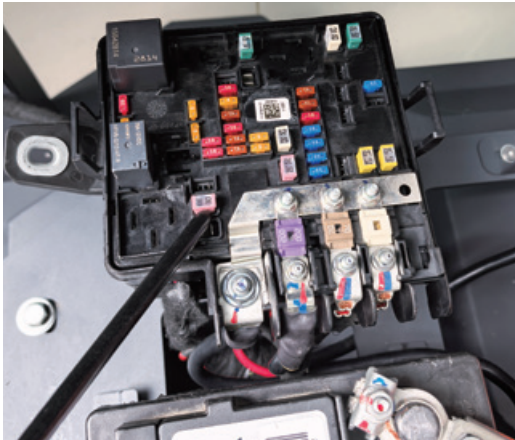
检测低速保险
