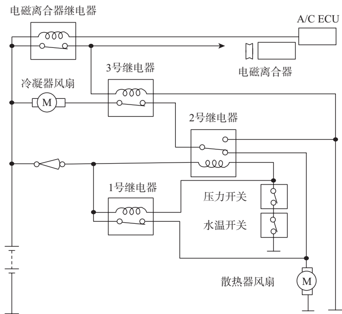
图 2-3-9 限流电阻式散热风扇控制电路
