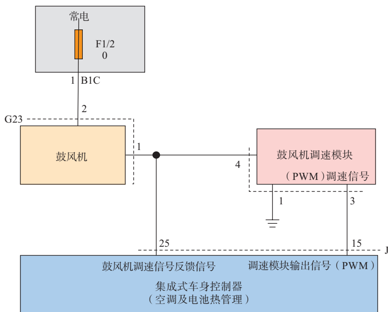
图 2-3-18 秦 PLUS EV 鼓风机电路
