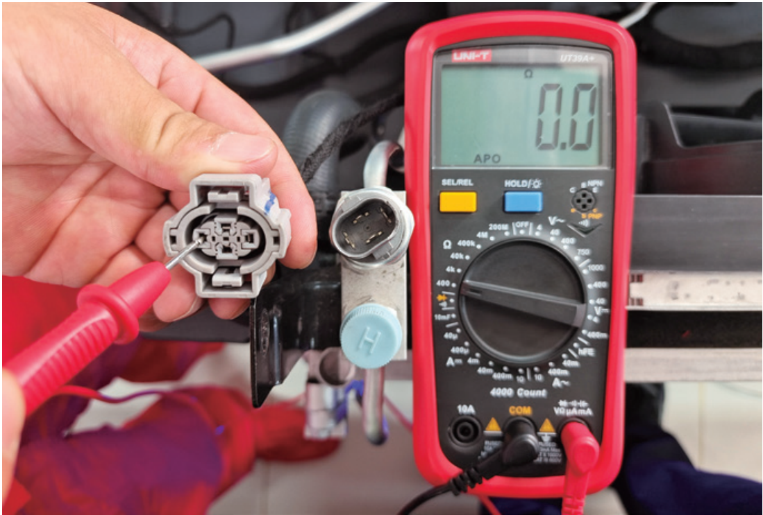
图 5-1-17 压力开关 2 号端子电压测量
