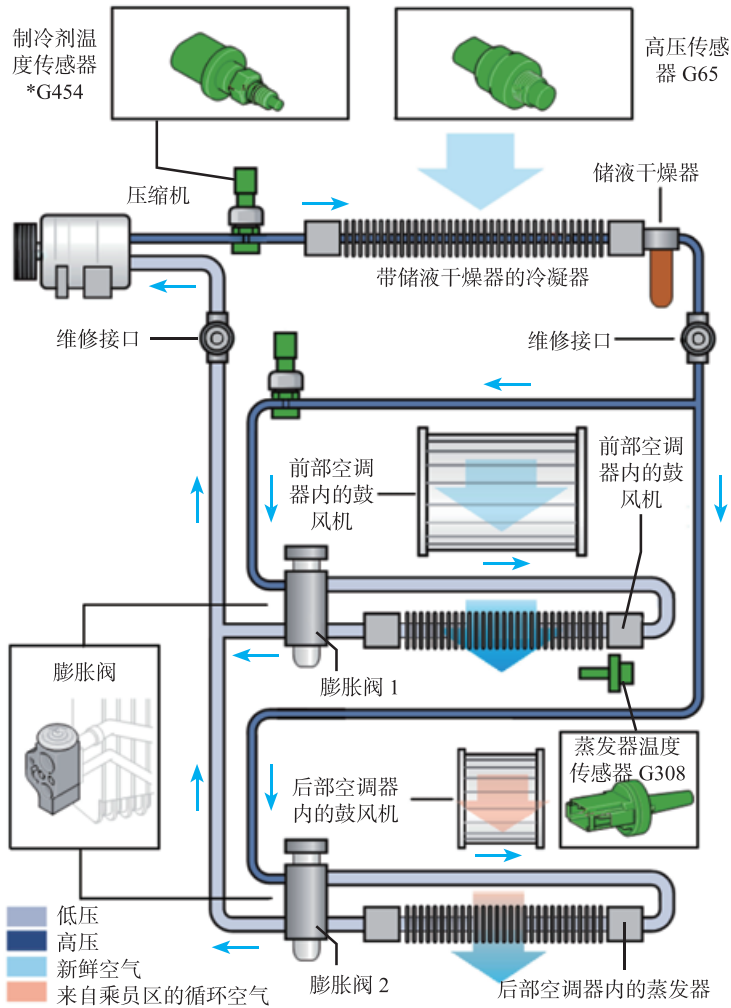
图 5-3-7 四温区空调制冷回路
