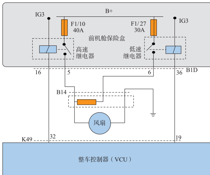
图 2-3-7 秦 PLUS EV 风扇控制电路
