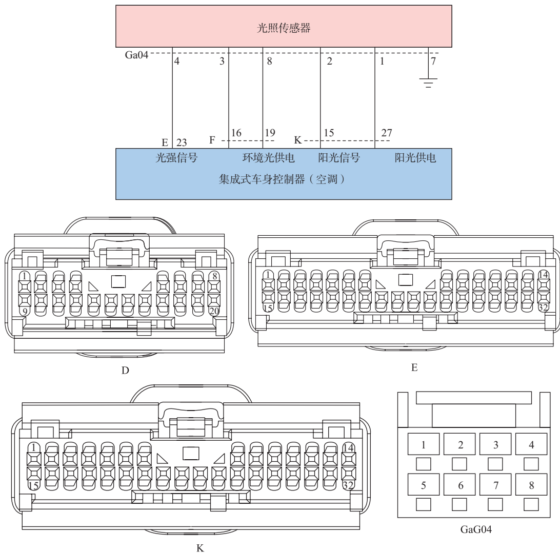
图 5-1-11 秦 PLUS EV 光照传感器电路及相关端子
