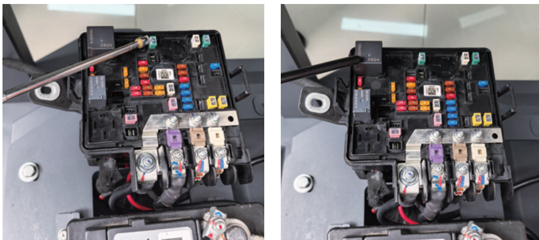
检测高速保险
