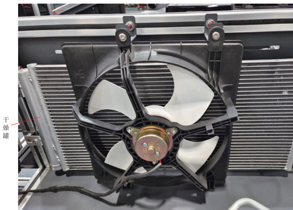
图 2-4-3 与冷凝器一体的储液干燥罐
