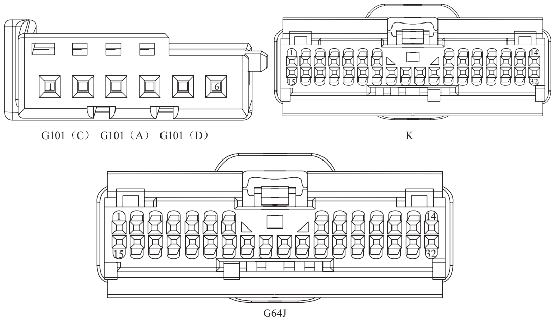
图 4-2-16 秦 PLUS EV 伺服电机端子
