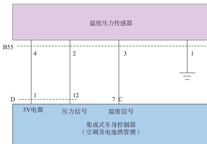
图 2-4-14 秦 PLUS EV 温度压力传感器电路
