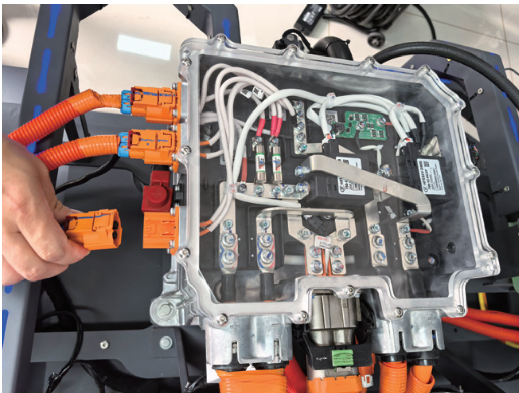
图 3-1-11 拔下空调暖风 PTC 的高压插头
