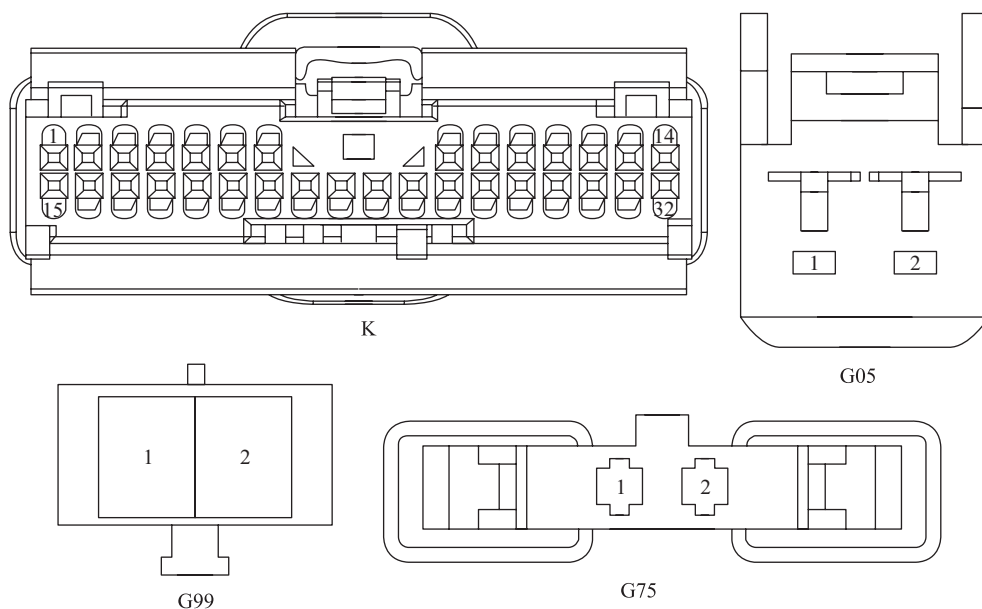
图 5-1-5 秦 PLUS EV 各车内温度传感器相关端子
