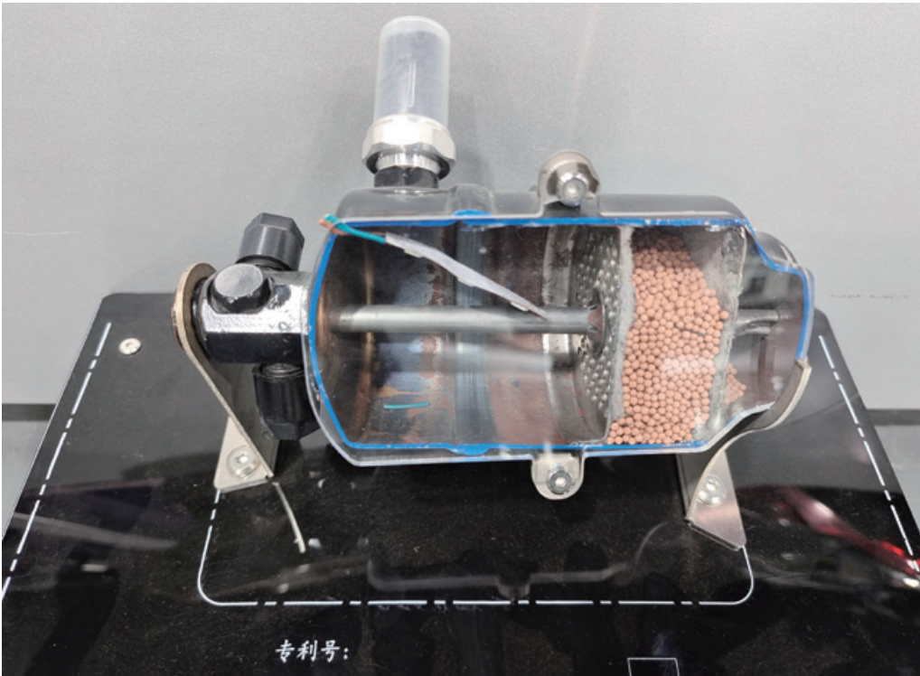
图 2-1-14 储液瓶干燥瓶
