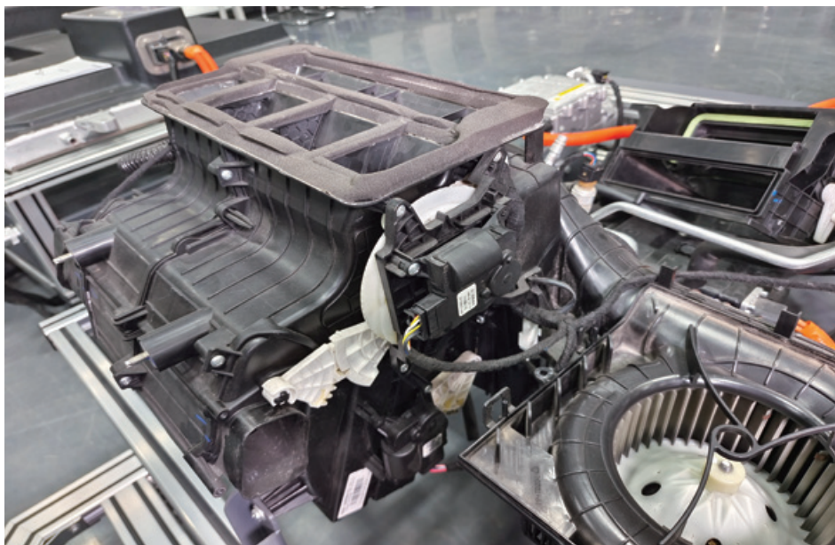
图 4-2-13 秦 PLUS EV 出风模式联动装置
