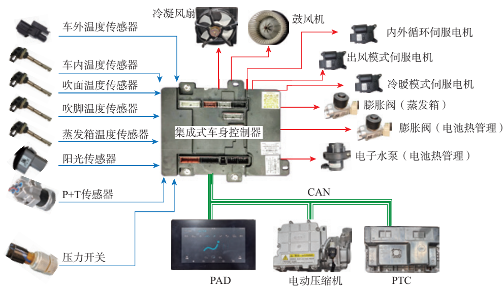
图 5-3-3 秦 PLUS EV 空调电路控制框架
