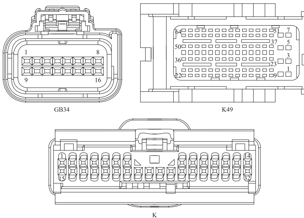
图 3-1-10 秦 PLUS EV PTC (空调) 相关插头
