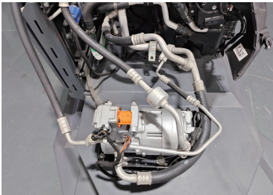
图 2-1-12 压缩机
