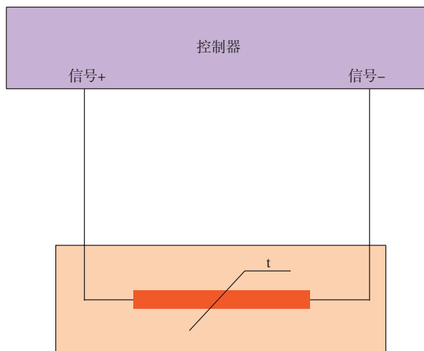
图 5-1-2 温度传感器电路
