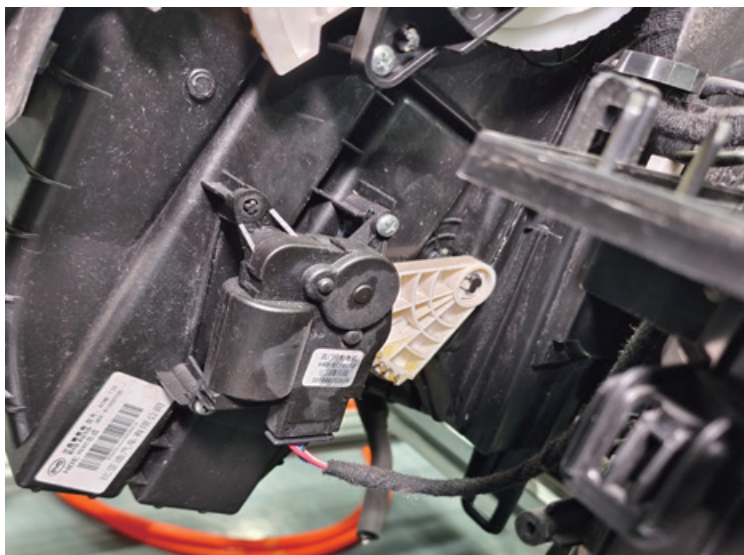
图 4-2-9 秦 PLUS EV 冷暖控制混合风门的控制
