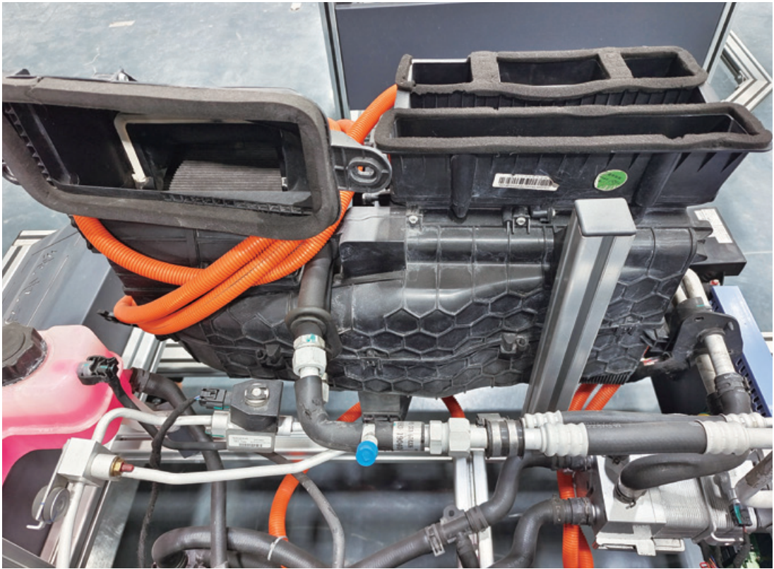
图 2-3-20 蒸发箱位置
