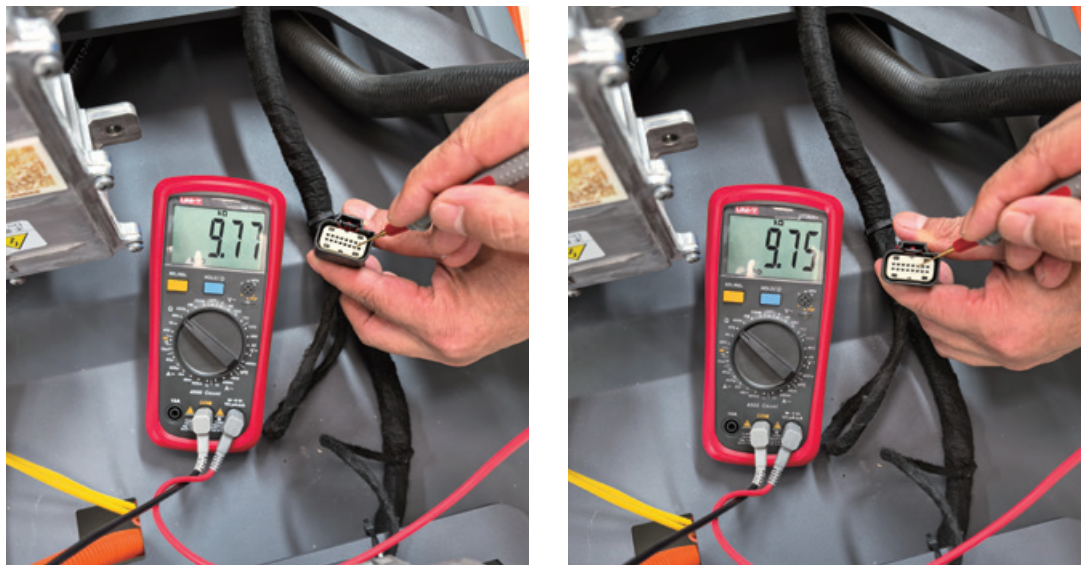
图 3-1-16 温度传感器测量
