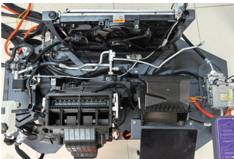
图 2-1-16 比亚迪秦 PLUS EV 空调系统
