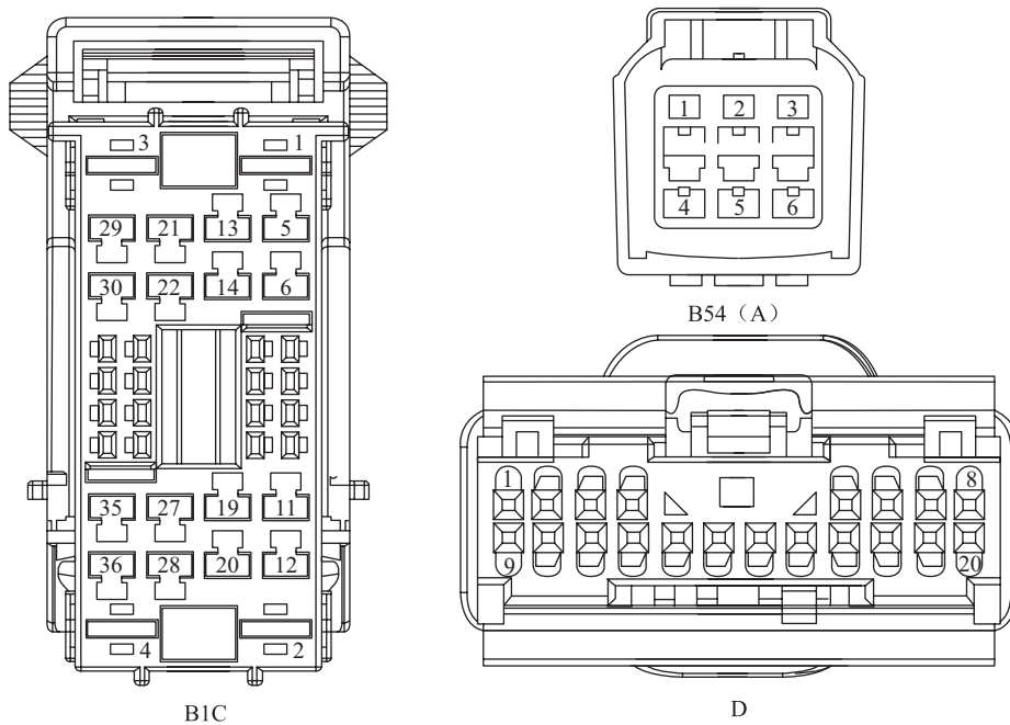
图 2-4-12 秦 PLUS EV 电子膨胀阀相关插头
