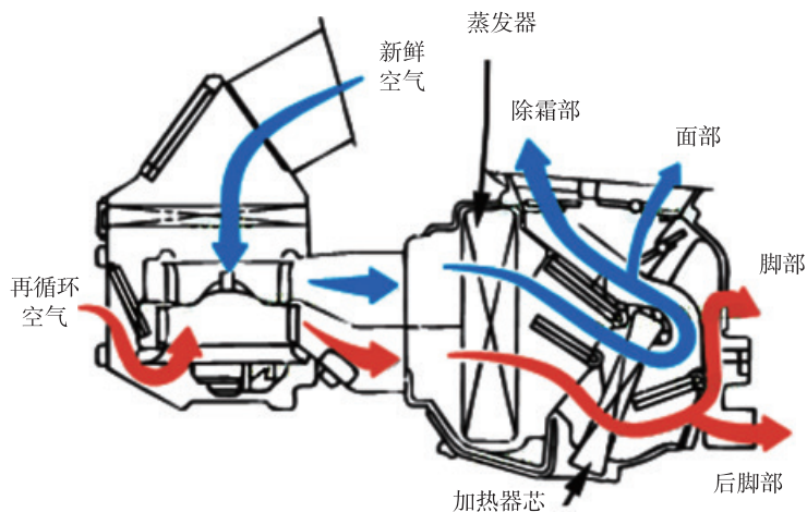
图 4-1-8 强制通风
