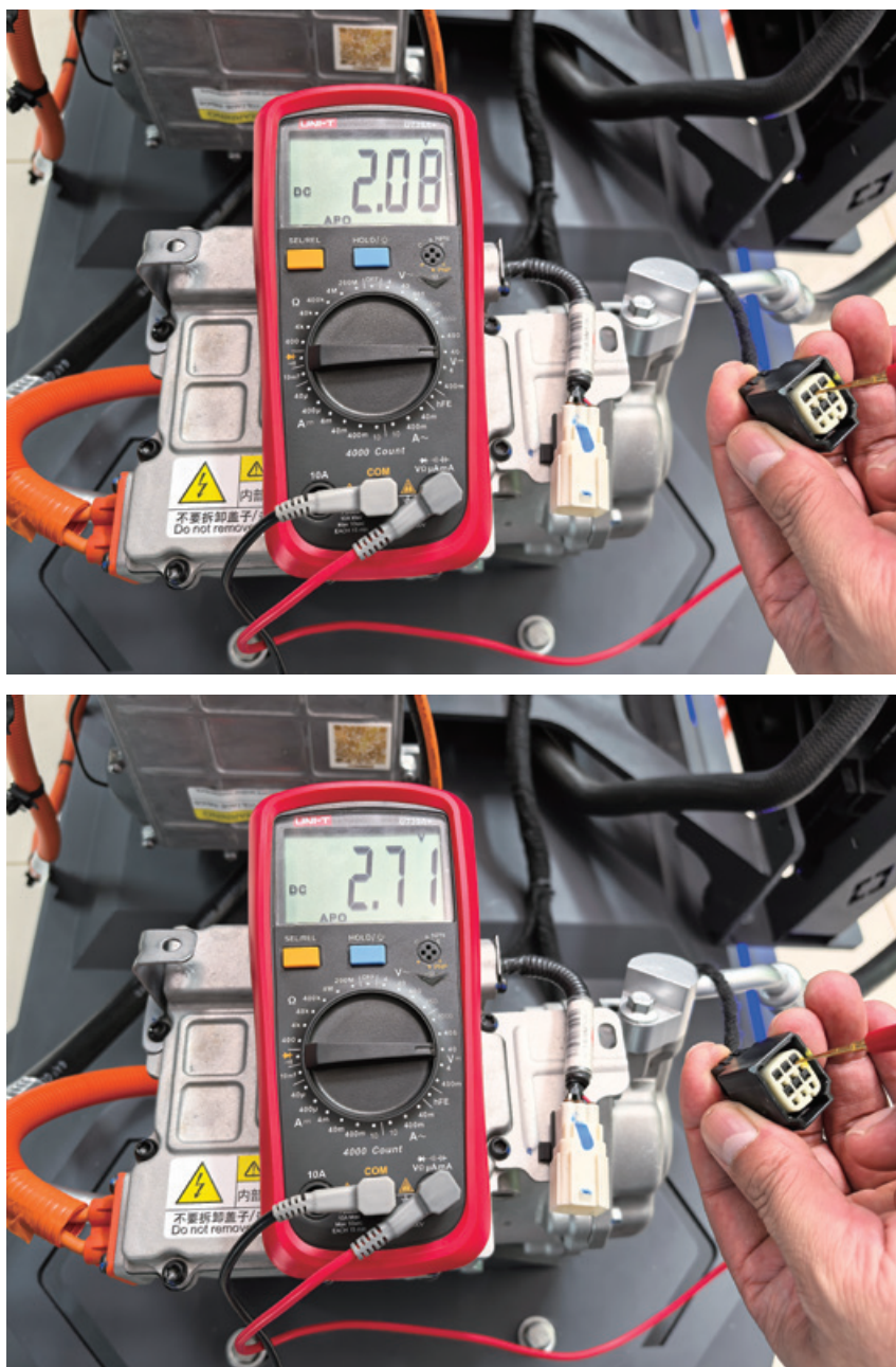
图 2-2-11 CAN 线信号测量
