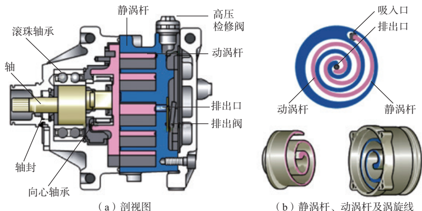
图 2-2-6 涡旋式压缩机构
