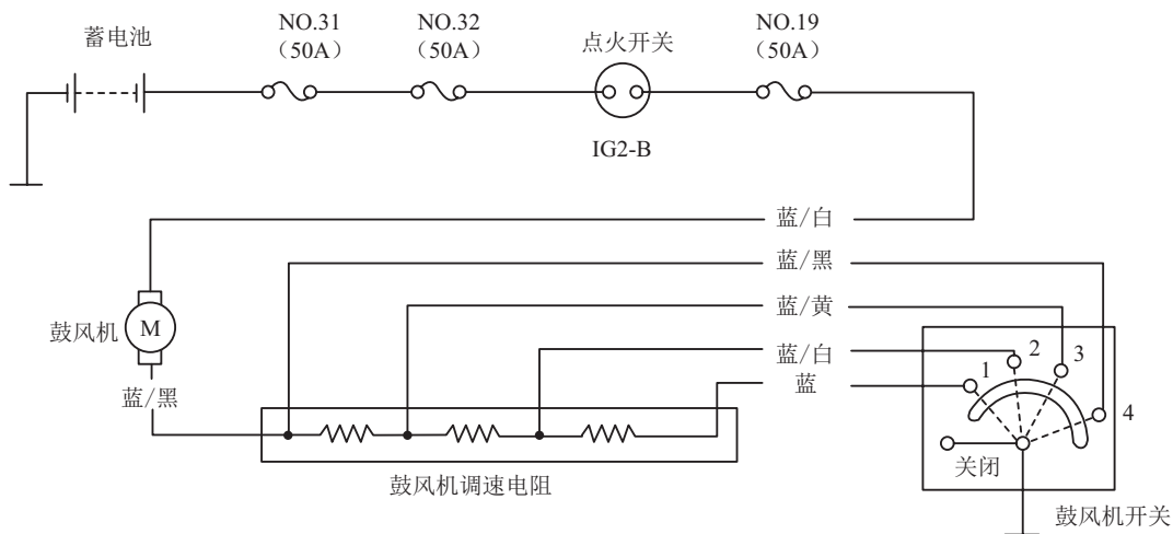
图 2-3-16 鼓风机串联电阻有级调速电路
