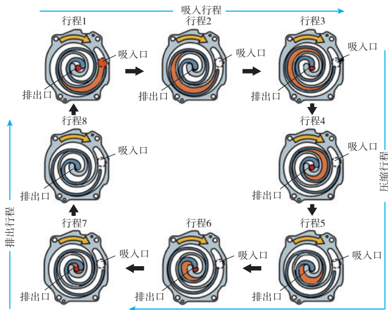
图 2-2-7 涡旋式压缩机的工作过程
