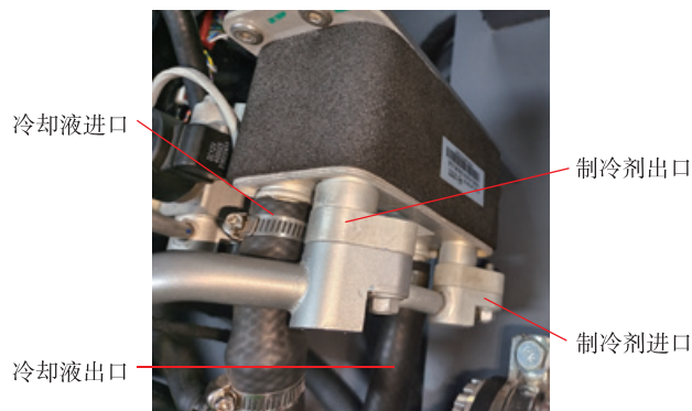
图 2-5-1 板式换热器
