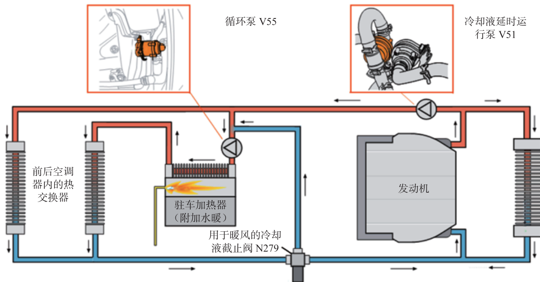
图 5-3-8 四温区空调制热回路
