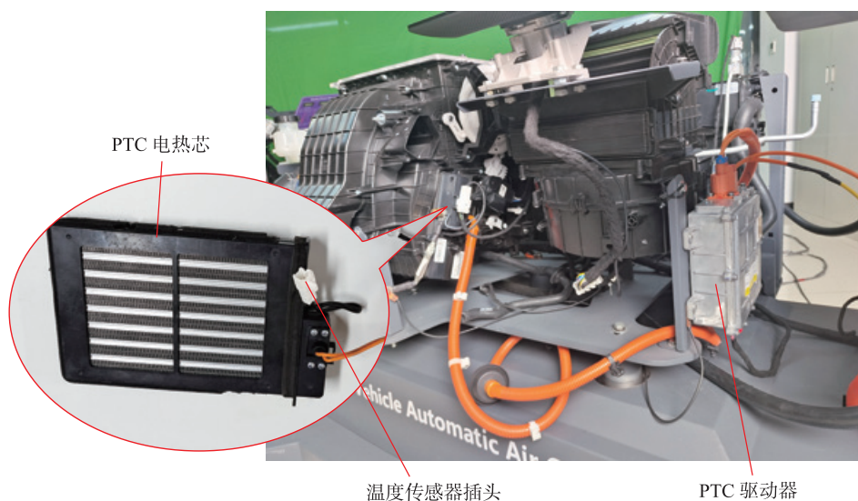
图 3-1-8 秦 PLUS EV 采用干式暖风系统
