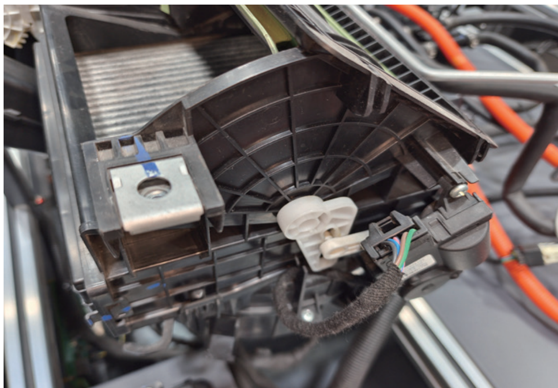
图 4-2-6 秦 EV 进气风门控制机构
