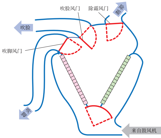
图 4-2-12 秦 PLUS EV 出风口风门控制示意图
