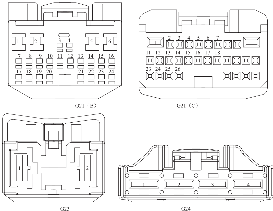
图 2-3-28 秦 EV 电动汽车鼓风机控制相关插头
