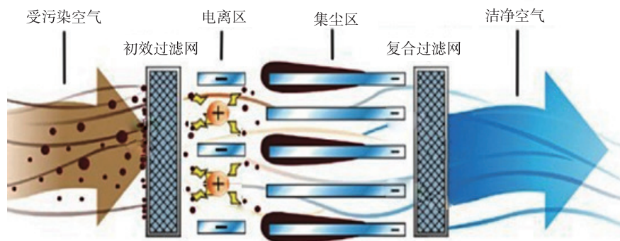
图 4-3-6 静电除尘净化系统的结构
