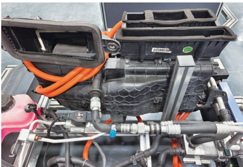
图 2-3-11 蒸发箱位置
