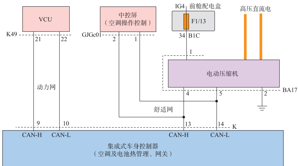
图 2-2-4 秦 PLUS EV 电动压缩机控制电路
