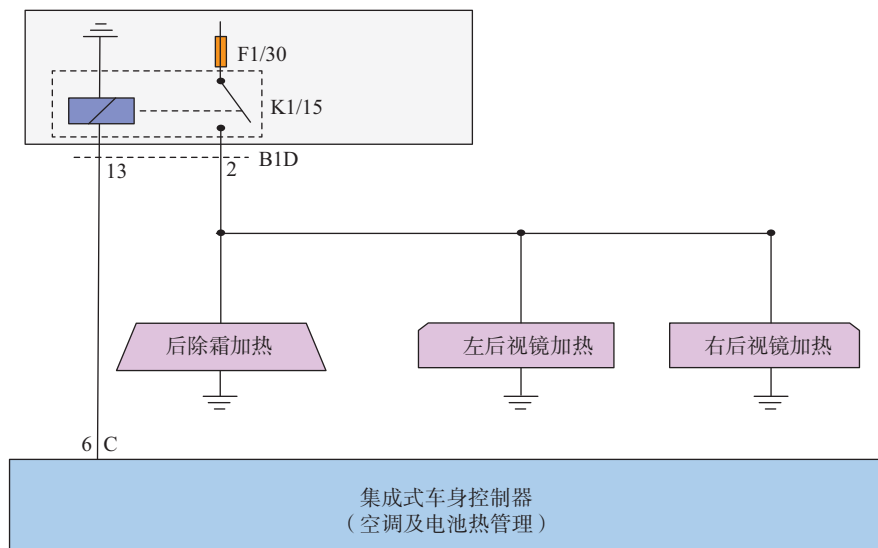
图 3-2-4 秦 PLUS EV 后风挡的除霜和倒车镜镜片的加热电路
