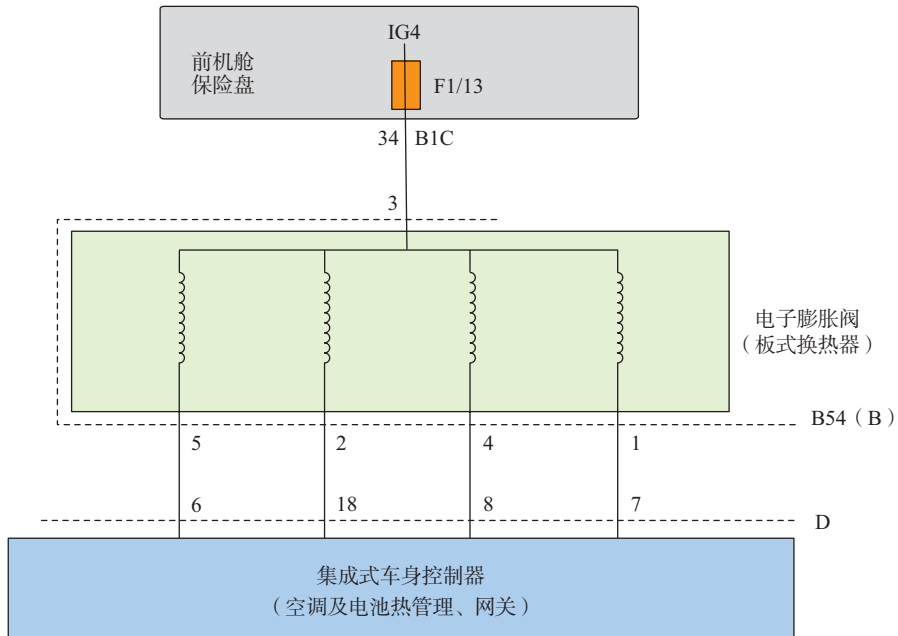
图 2-5-4 板式换热器的电子膨胀阀电路
