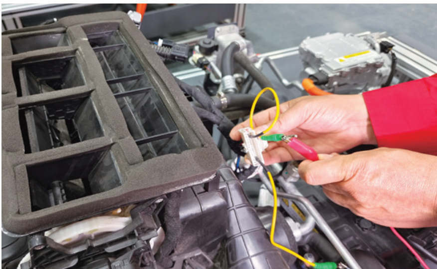
图 4-2-22 出风模式风门伺服电机通电实验（转向除霜端）
