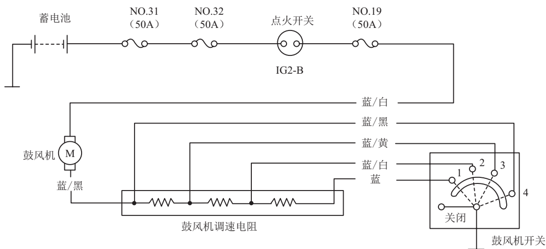
图 2-3-25 鼓风机串联电阻有级调速电路
