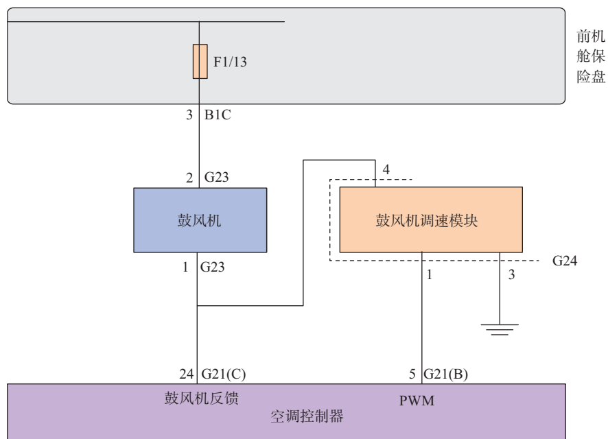
图 2-3-27 秦 EV 电动汽车鼓风机控制电路
