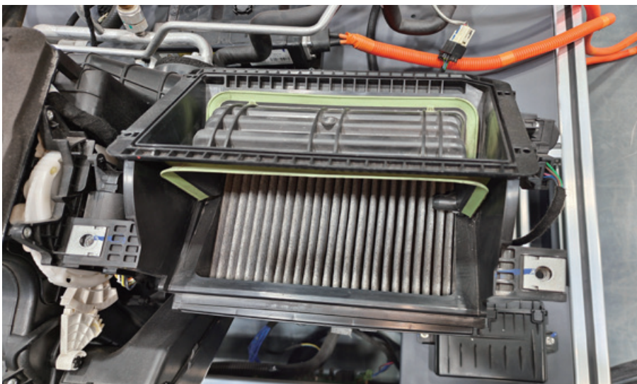
图 4-2-4 秦 PLUS EV 进风口
