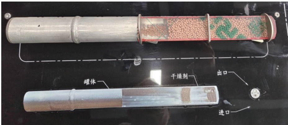
图 2-4-4 与冷凝器一体式储液干燥罐内部结构
