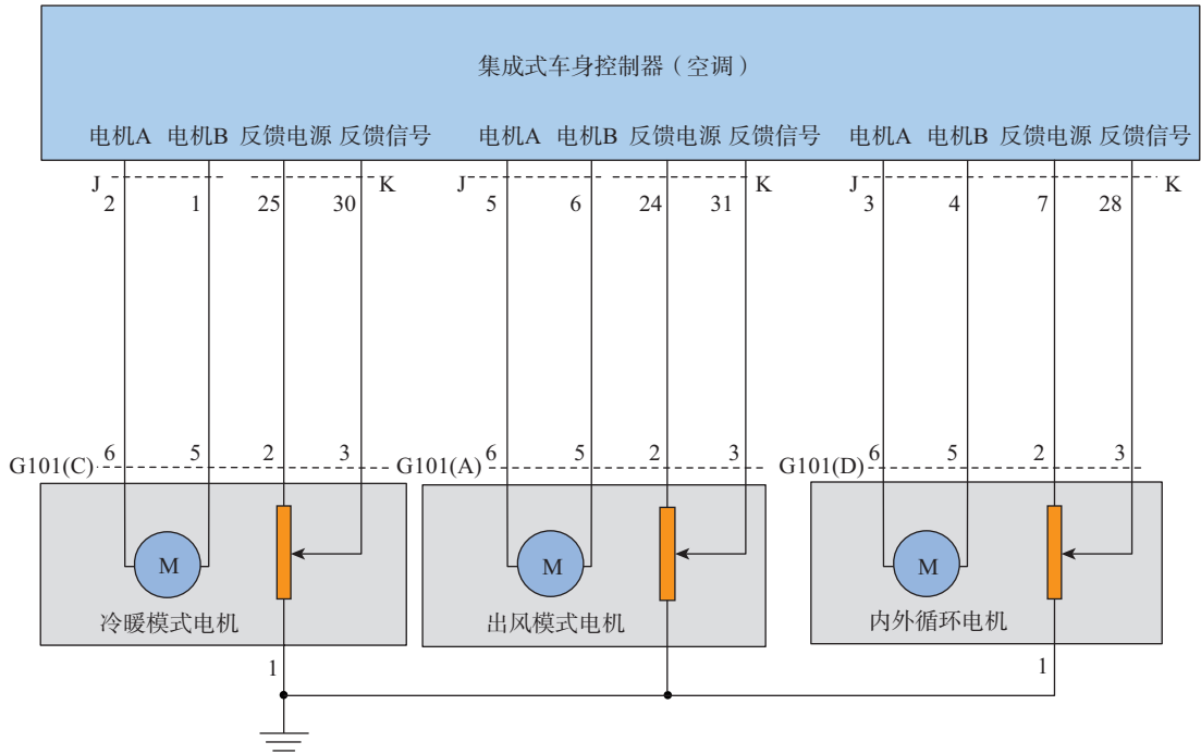
图 4-2-15 秦 PLUS EV 伺服电机电路
