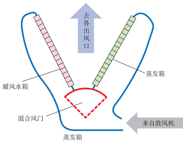
图 5-2-8 温度调节旋钮中间时冷暖空气混合风门位置
