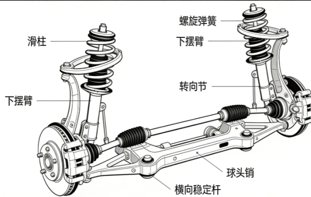
麦弗逊式独立悬架结构图
